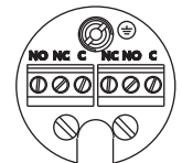
CONEXIONES TERMINAL DPDT
